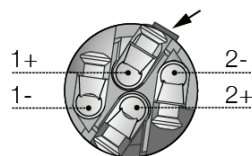
NL4 input/output wiring
